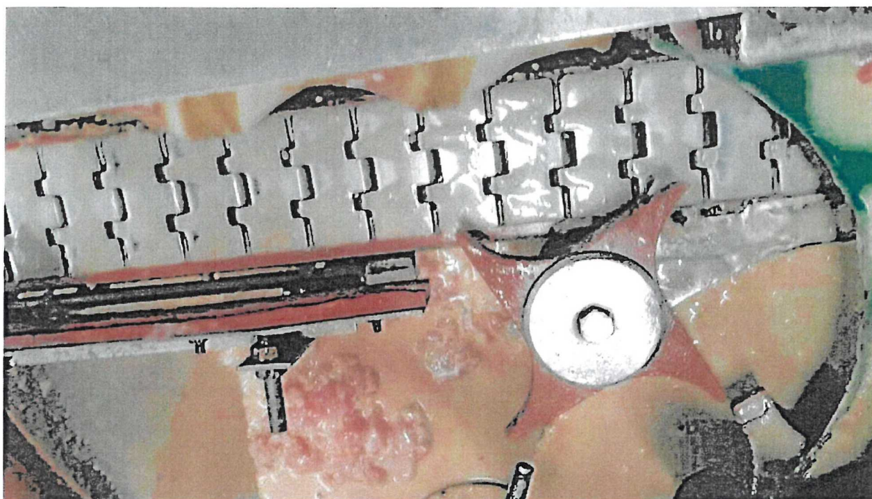
Obrázek 5 - Plnicí stroj omáček „PLAO“ - pohled na část šneku, na dopravník, a na celou podávací hvězdu, která přisunuje plněné obaly do plnicího karuselu.
