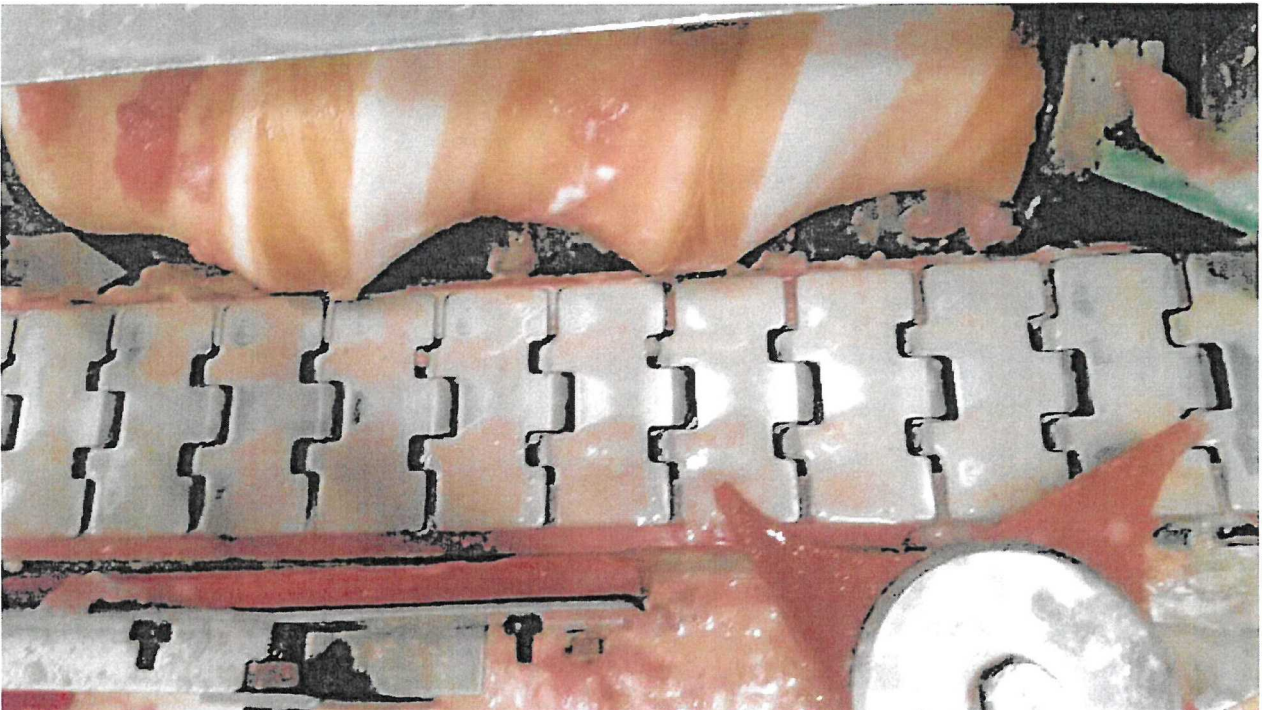
Obrázek 4 - Plnicí stroj omáček „PLAO“ - pohled na šnek, na dopravník a na část podávací hvězdy.
