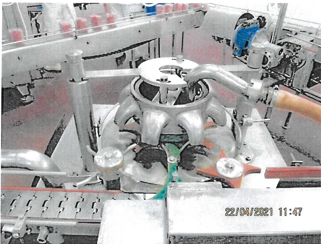
Obrázek 1 - Celkový pohled na vyčištěný Plnicí stroj omáček „PLAO“ pořízený dne 22.04.2021.
