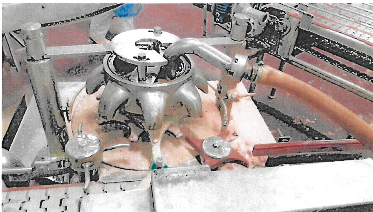
Obrázek 2 - Celkový pohled na Plnicí stroj omáček „PLAO“ - stav stroje po úrazu [REDACTED]
